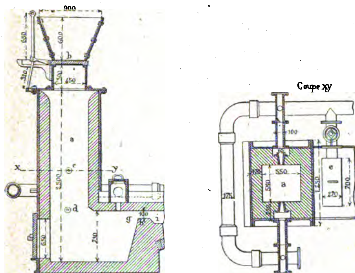
Fig. 103-104. — Gazogène à flamme renversée.
